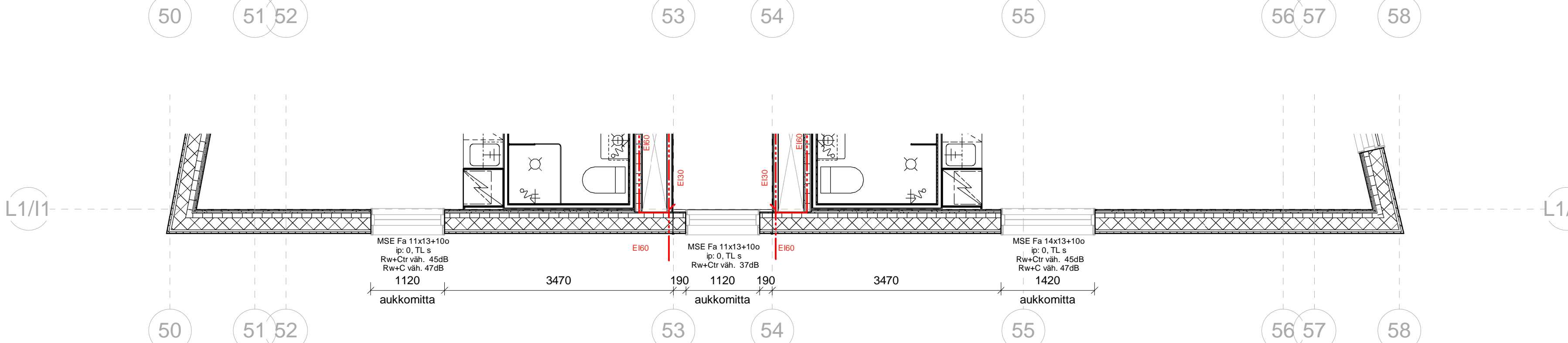
kerrokset 6-8, eteläpääty 1 : 50
