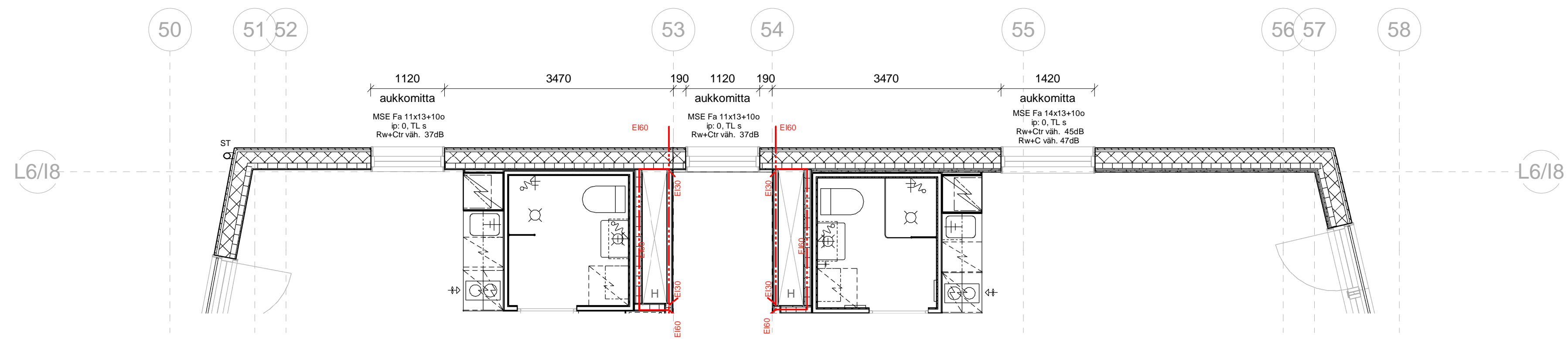
kerrokset 6-8, pohjoispääty 1 : 50
