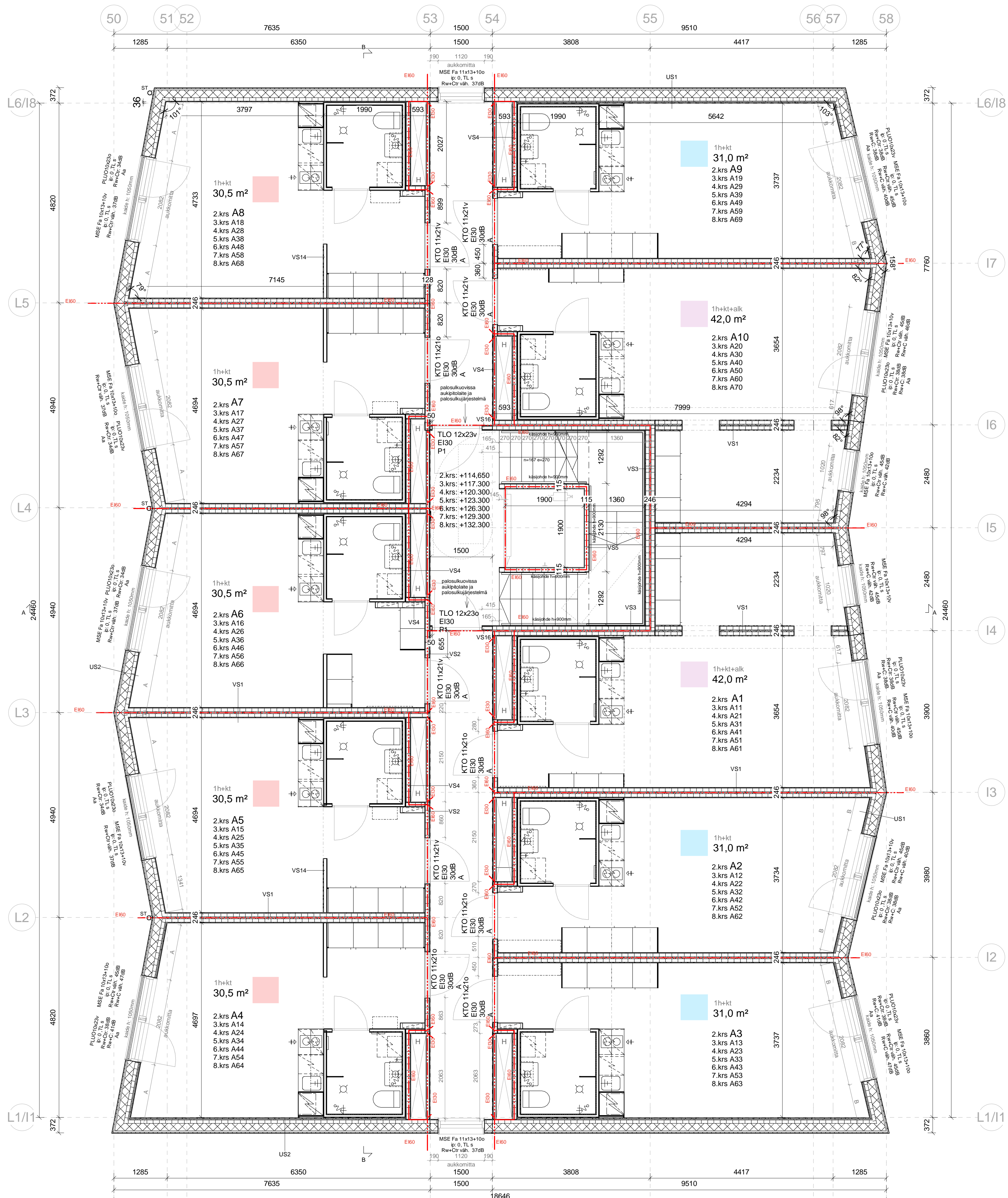
KERROKSET 2-8 1 : 50
