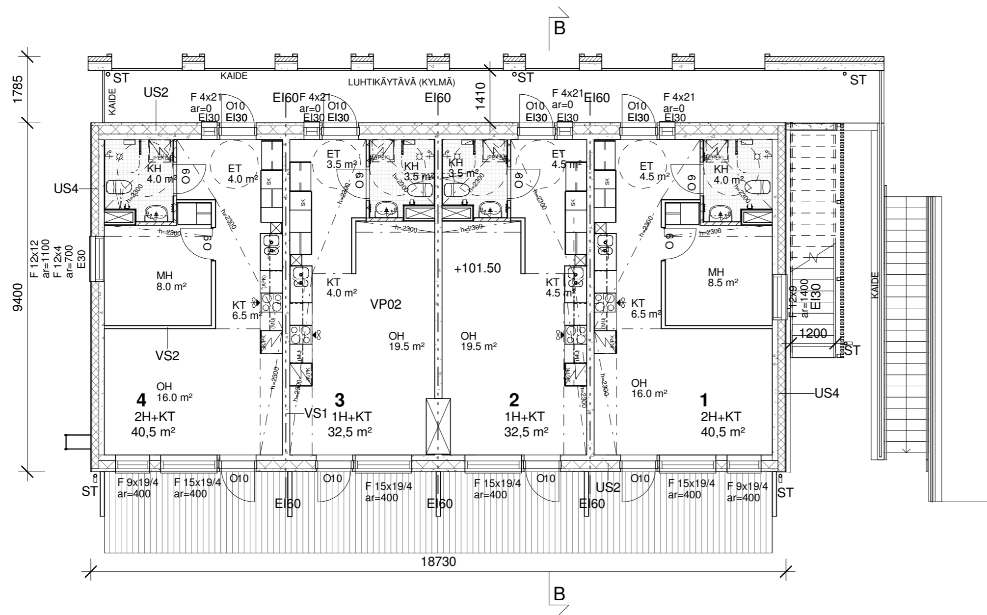
2. kerros 1 : 100
