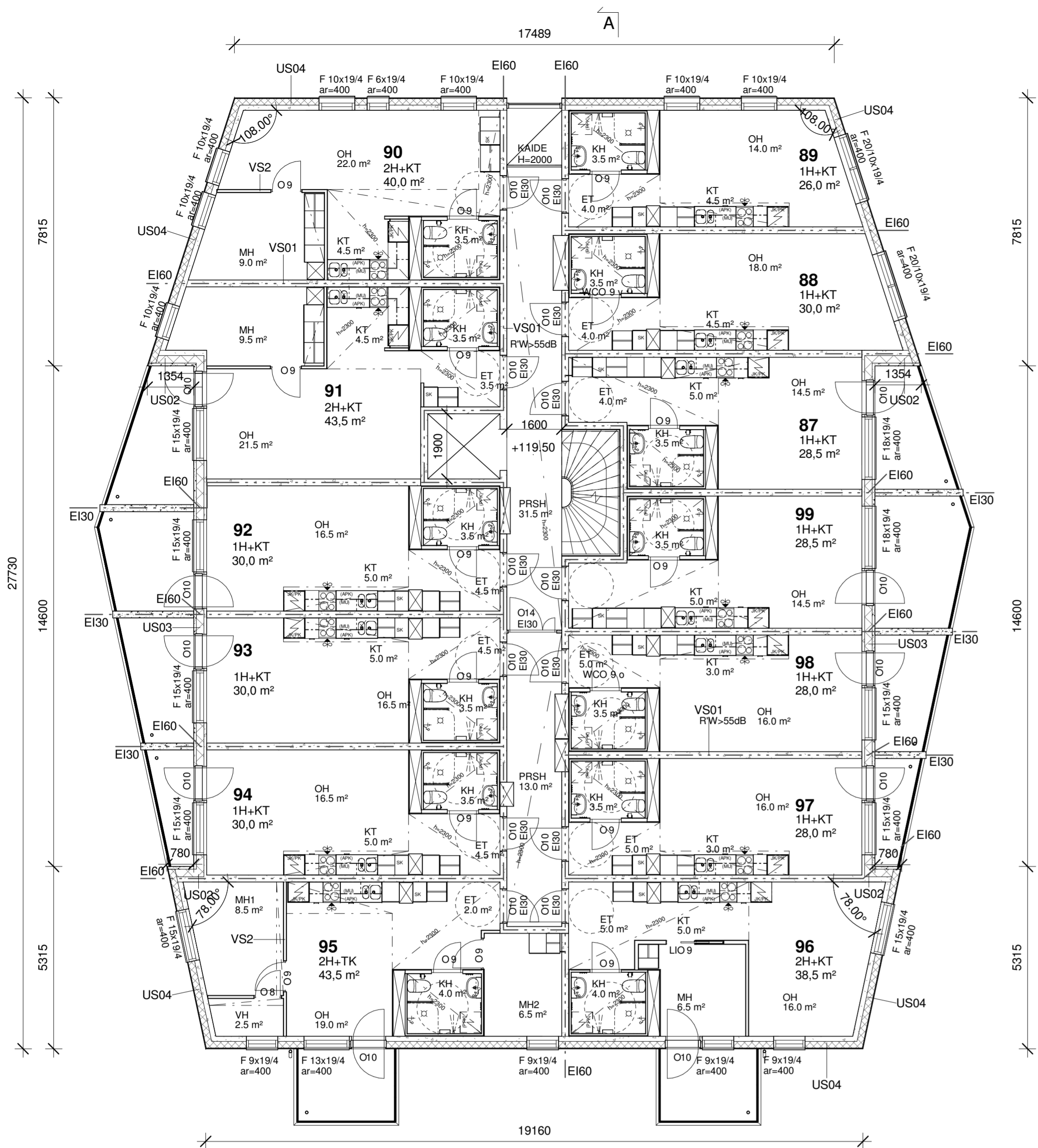
8. kerros 1 : 100
