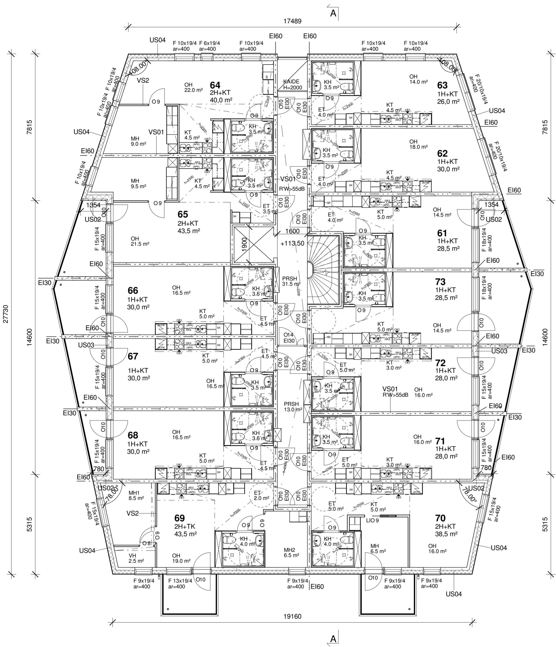
6. kerros 1 : 100
