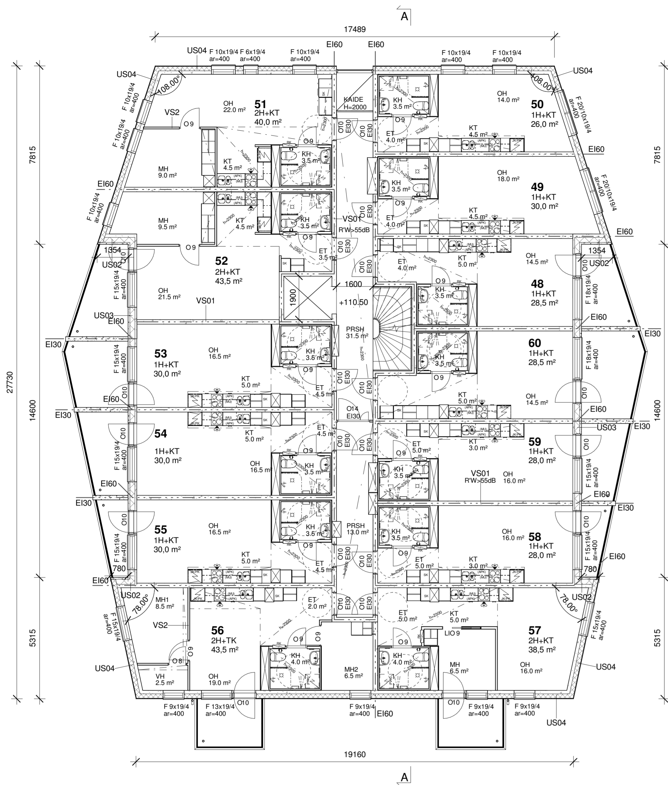
5. kerros 1 : 100
