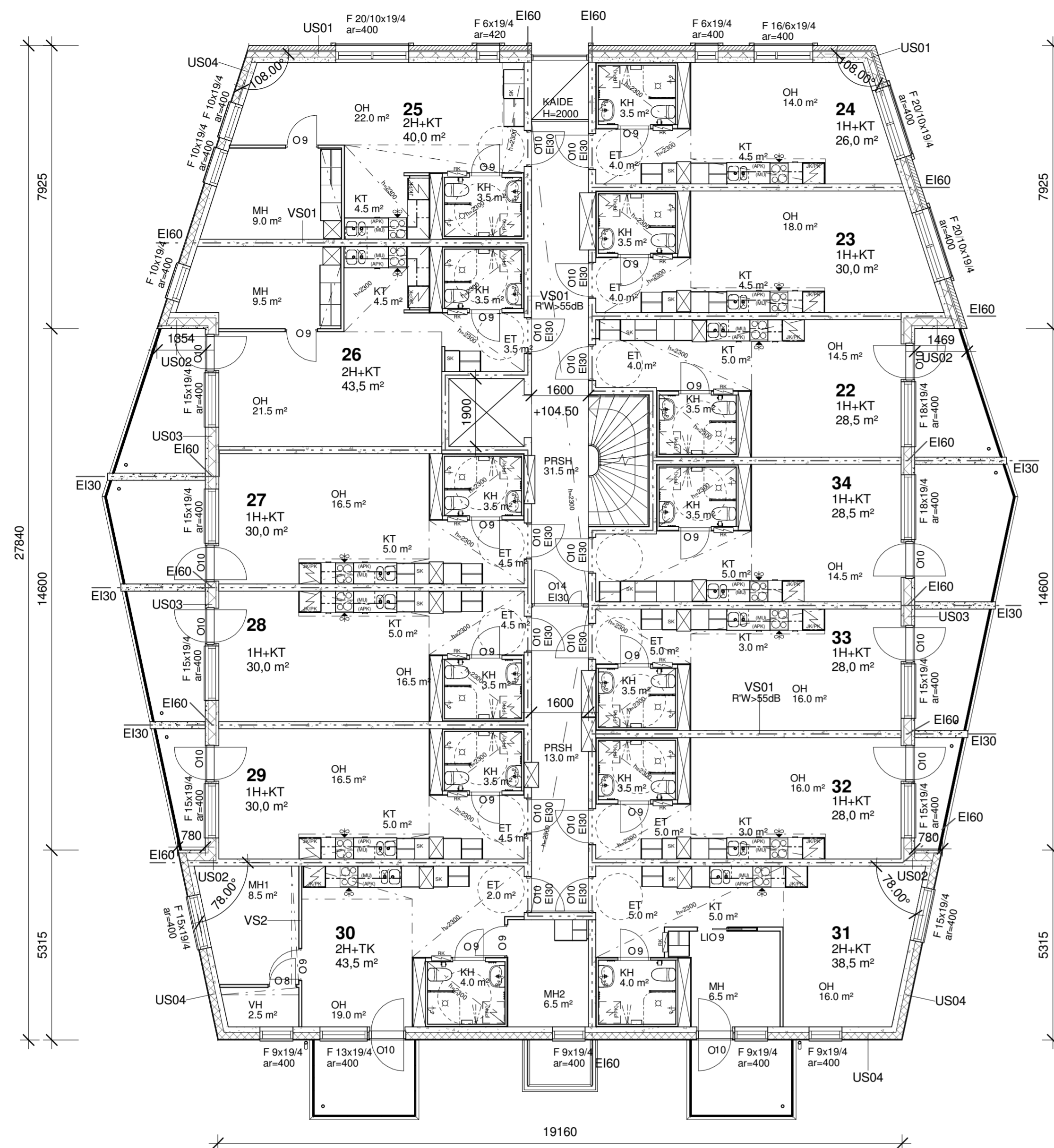
3 kerros 1 : 100
