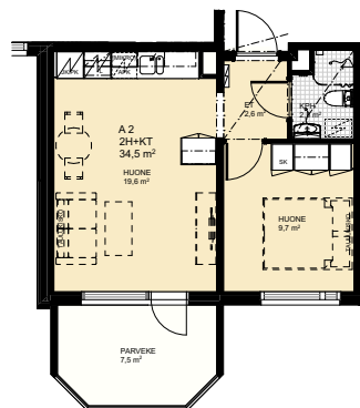
Huoneistotyyppi 2H+KT+P 34,5 m 2
