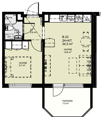
Huoneistotyyppi 2H+KT+P 34,5 m 2
