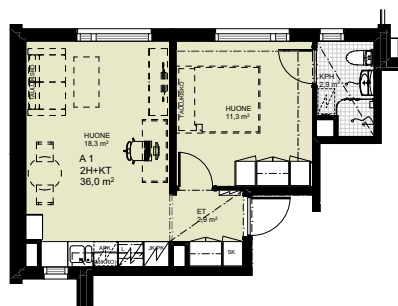
Huoneistotyyppi 2H+KT 36,0 m 2
