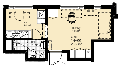
Huoneistotyyppi 1H+KK 23,5 m 2
