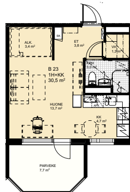
Huoneistotyyppi 1H+KK+P 30,5 m 2
