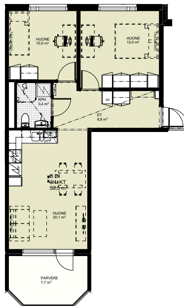
Huoneistotyyppi 3H+KT+P 56,5 m 2
