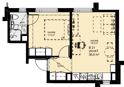
Huoneistotyyppi 2H+KT 36,0 m 2
